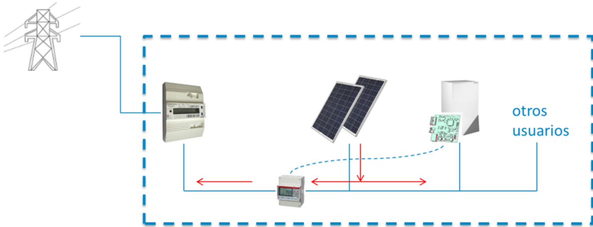
Figura 6. Sistema conexión Red Fotovoltaica.
