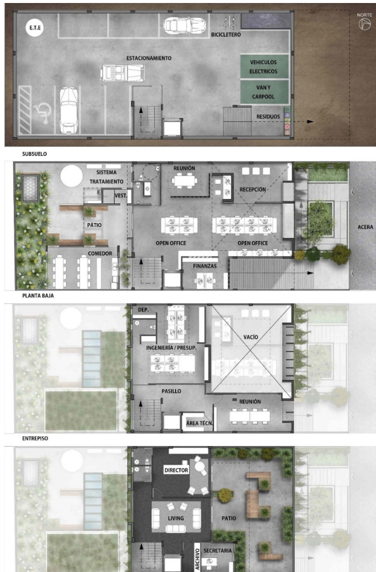
Figura 2. Plantas de la edificación.
